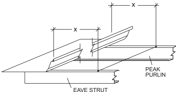
EAVE STRUT
